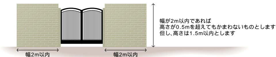
門及び門袖
